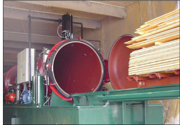
Mynd 1. Gagnvarnartankur.
